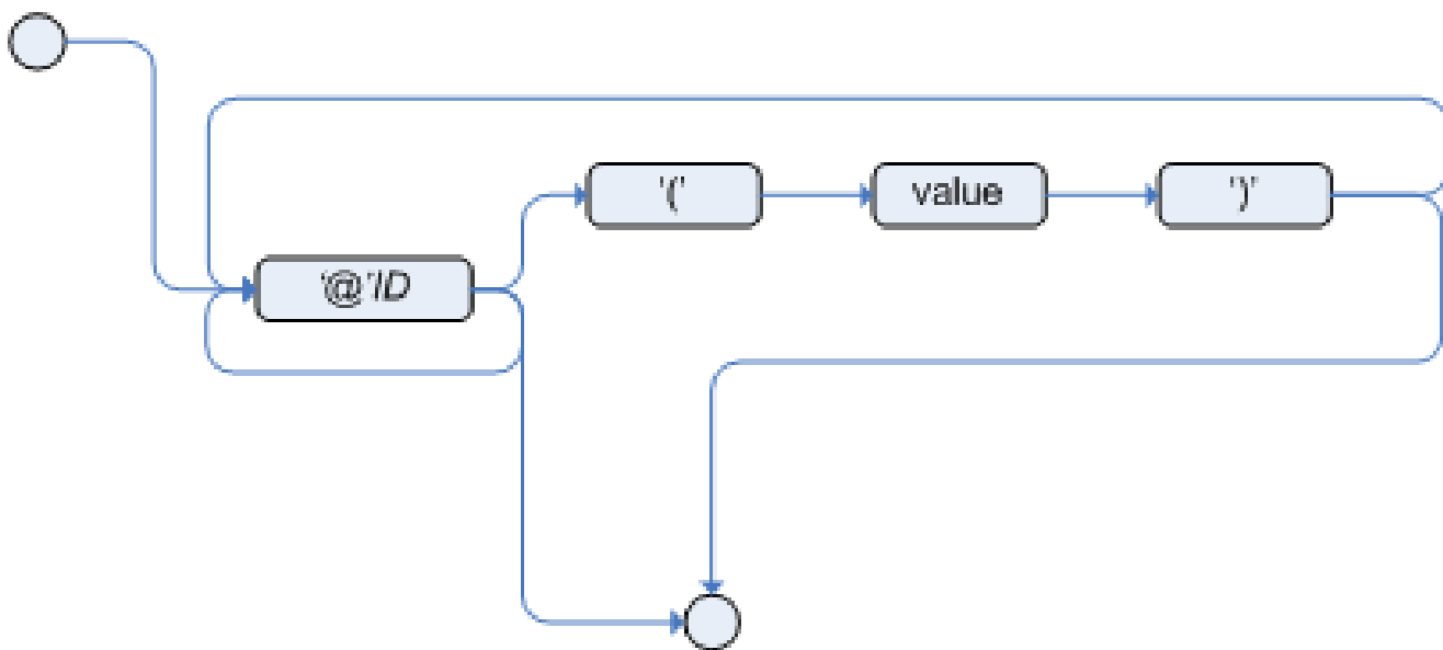
Figure 5.8. meta_data
