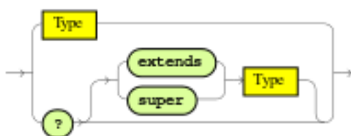
TypeArgument
