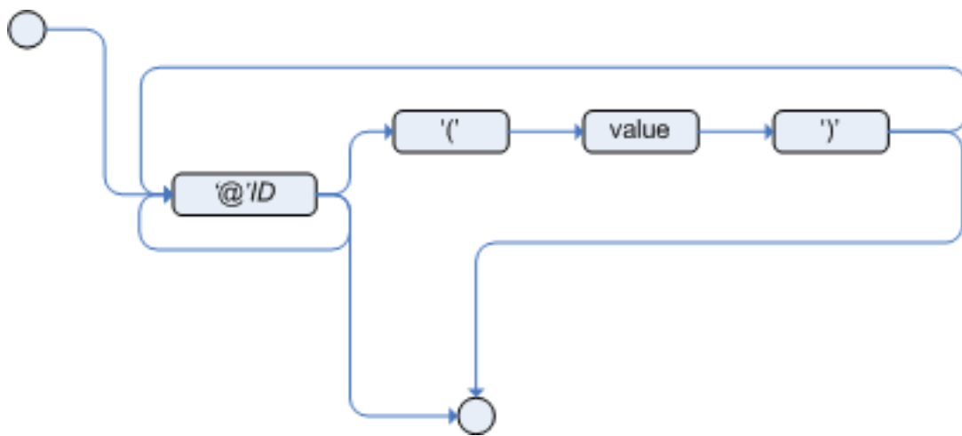
Figure 8.7. meta_data
