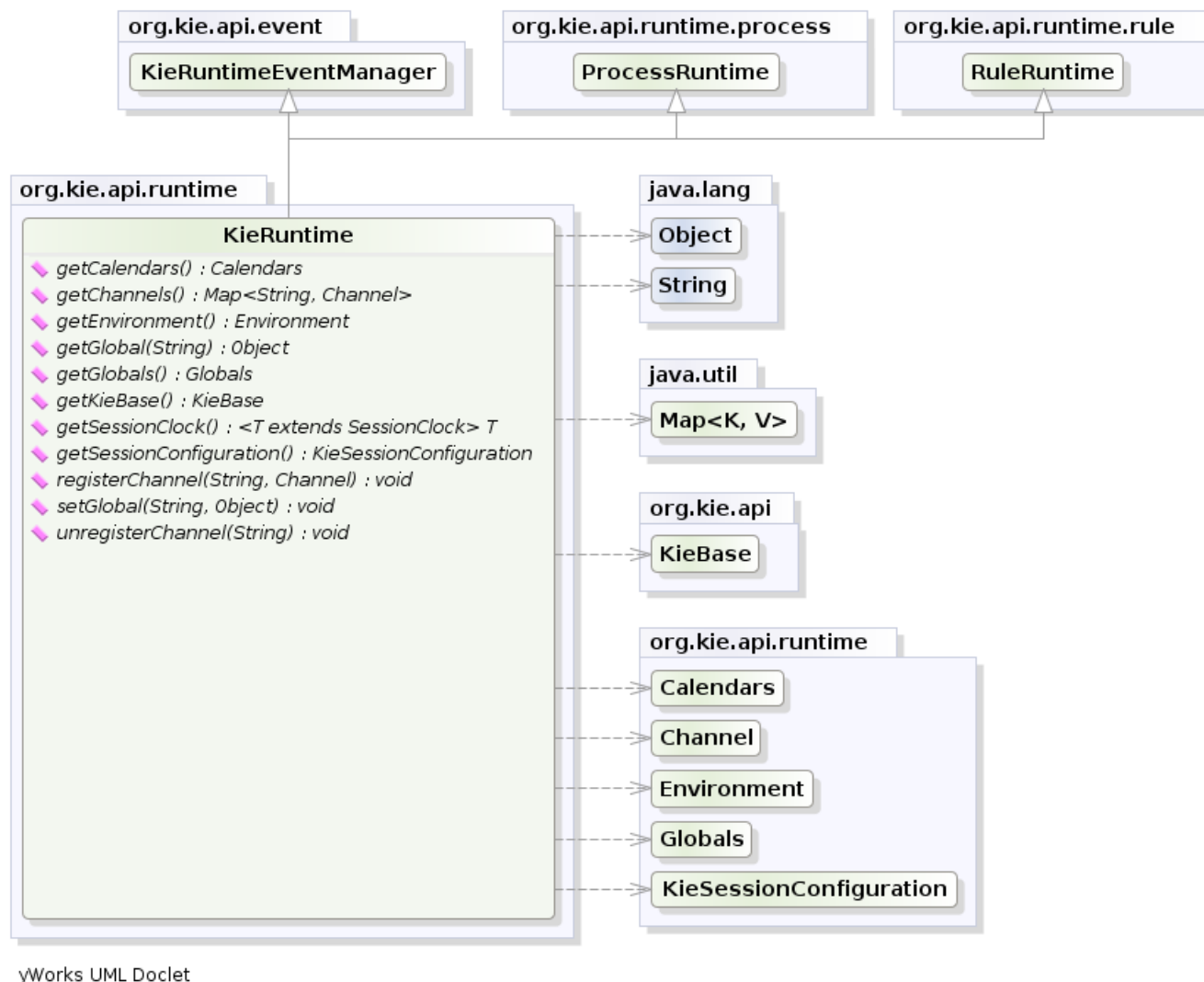
Figure 4.17. KieRuntime
