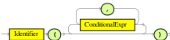
AccumulateInit
